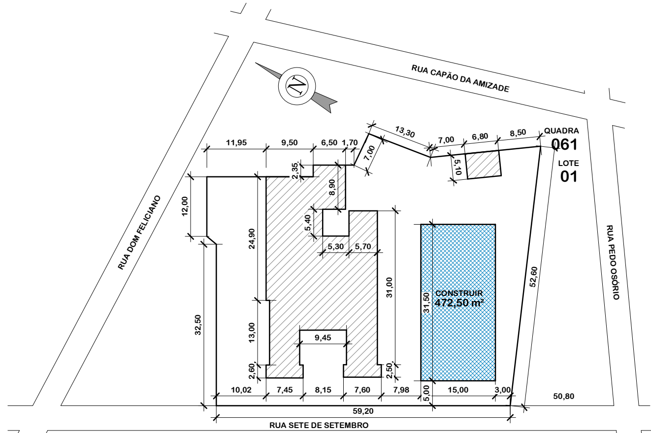
SITUAÇÃO/LOCALIZAÇÃO Esc.: 1 : 750
