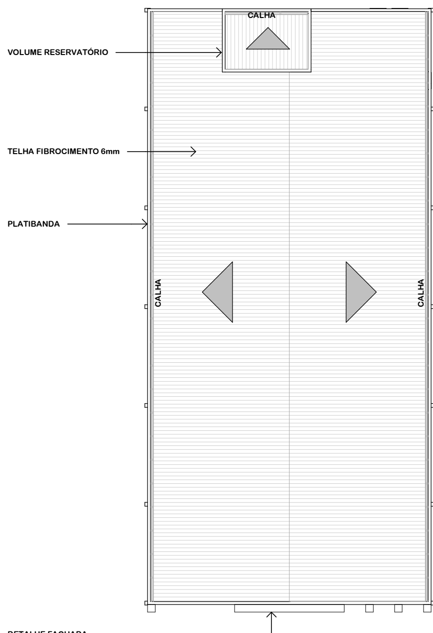
COBERTURA Esc.: 1 : 200
